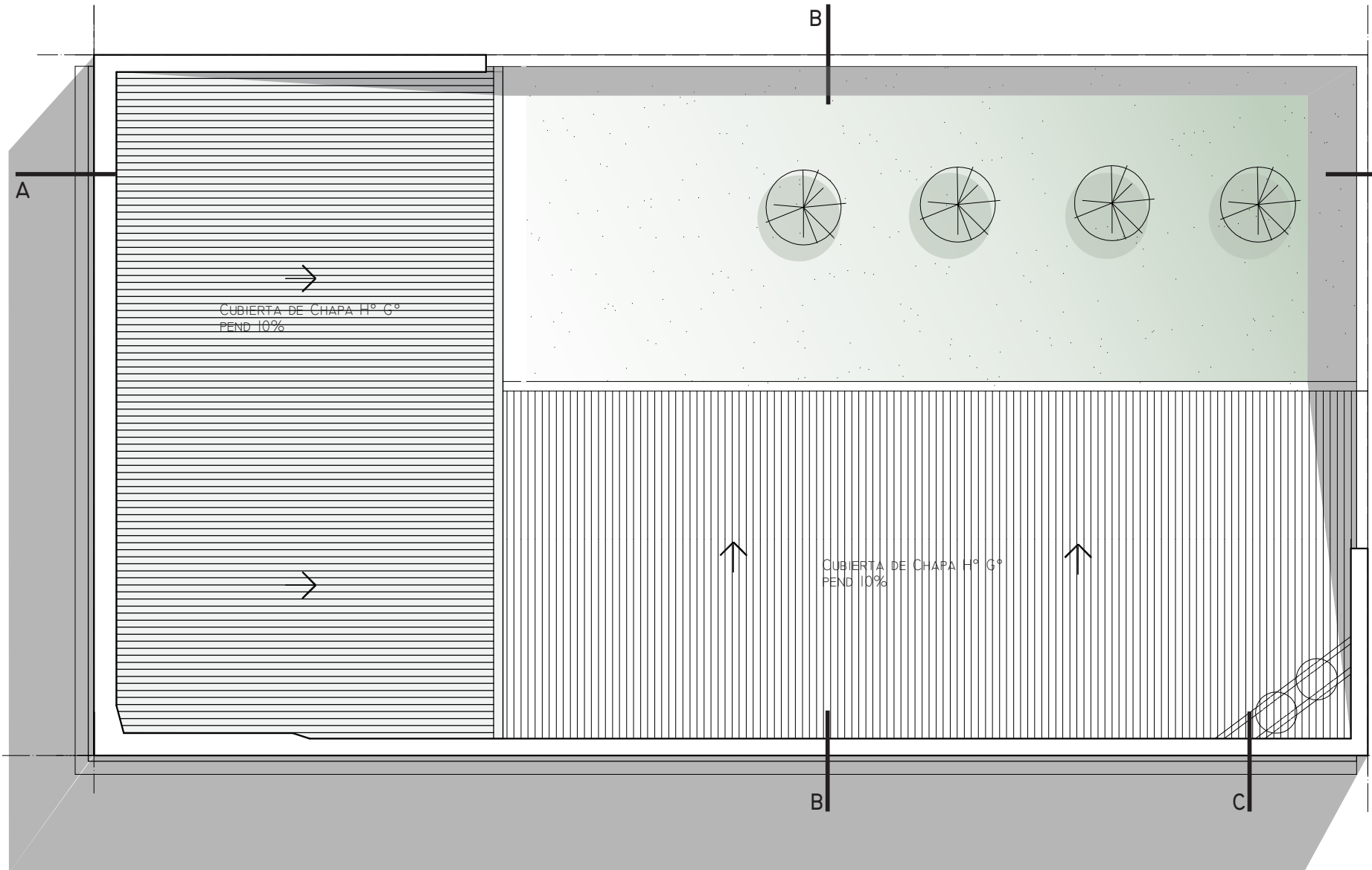
PLANTA CUBIERTA GENERAL
